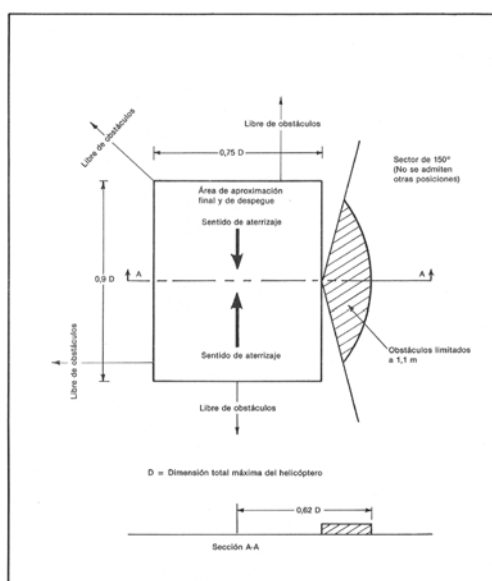
Figura 4-5H. Sectores limitadores de obstáculos en la heliplatforma Helicópteros de rotor principal en tándem - Operaciones bidireccionales
