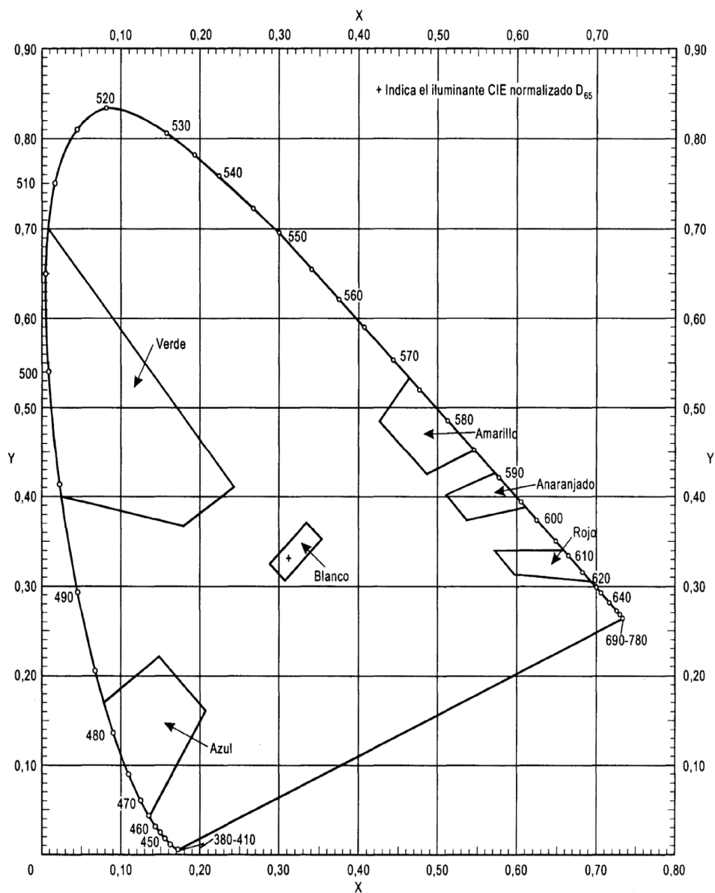
Figura A1 - 3. Colores de los materiales retrorreflectantes para las señales, letreros y tableros
