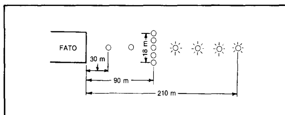
Figura 5-10H. Sistema de luces de aproximación
