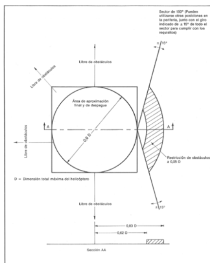
Figura 4-4H. Sectores limitadores de obstáculos en la heliplatforma Helicópteros de rotor principal en tándem - Operaciones omnidireccionales
