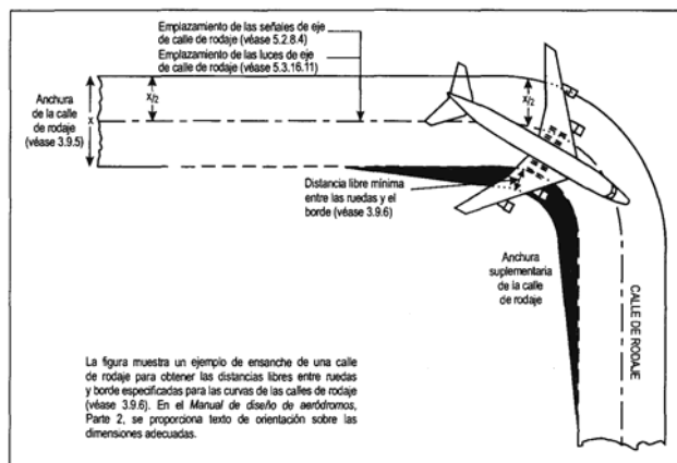
Figura 3 - 2. Curva de calle de rodaje
